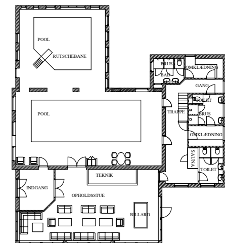
STUEPLAN
